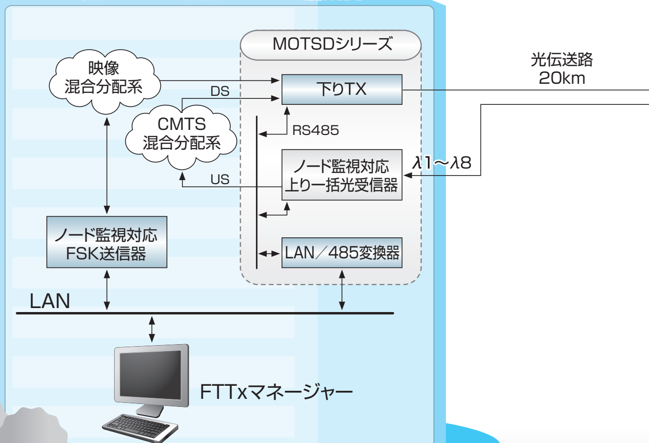
光センター装置システム構成例
